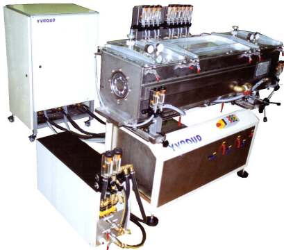
Ensemble de coextrusion pour tubes multi-couches
