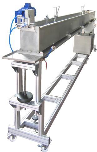
Bac par immersion 6 m type BAI6000-C avec convoyeur immergé et circuit fermé
